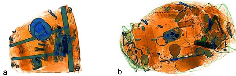
Abbildung 7 Röntgenbilder von zwei Gepäckstücken. a Das Gepäck auf der linken Seite ist ungefährlich. b Im Gepäck rechts ist eine Pistole und ein Messer enthalten.
