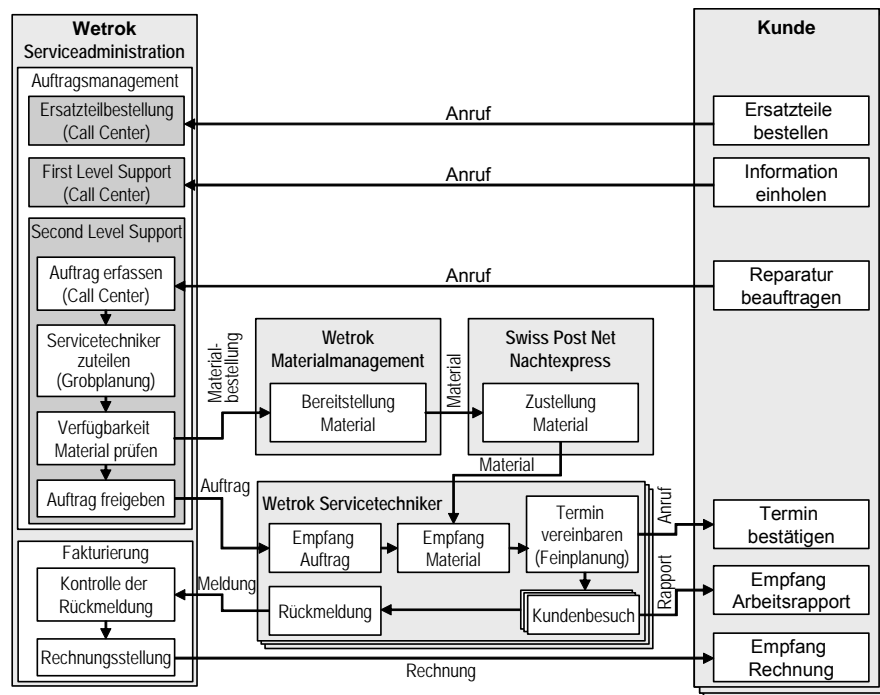
Abb. 21.1: Prozessübersicht der Serviceleistungen bei Wetrok
