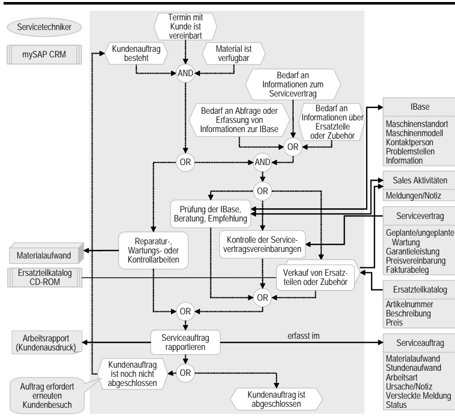
Abb. 21.2: Detailprozess Kundenbesuch des Servicetechnikers
