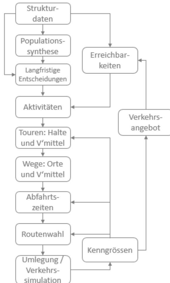
Abb. 15 Allgemeine Modellstruktur eines aktivitätsbasierten Verkehrsmodells
