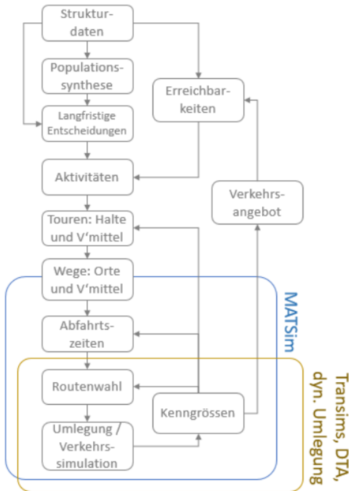
Abb. 19 Allgemeine Datenstrukturen von aggregierten und aktivitätenbasierten Verkehrsmodellen
