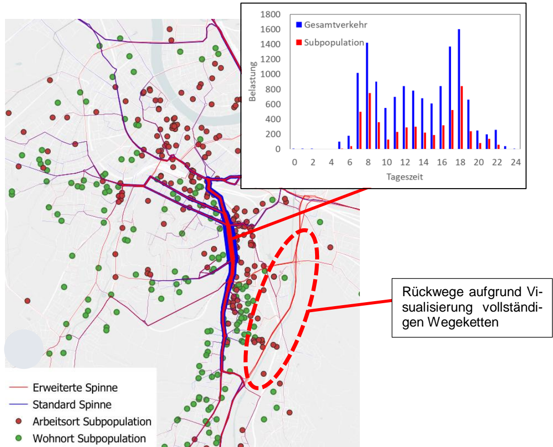
Abb. 52 Querschnittsbelastung mit einer erweiterten Spinne, welche die ganzen Wegeketten abbildet, und Tagesganglinie, inklusive Auswertung einer ausgewählten Subpopulation (hier 25-64 Jahre, männlich).
