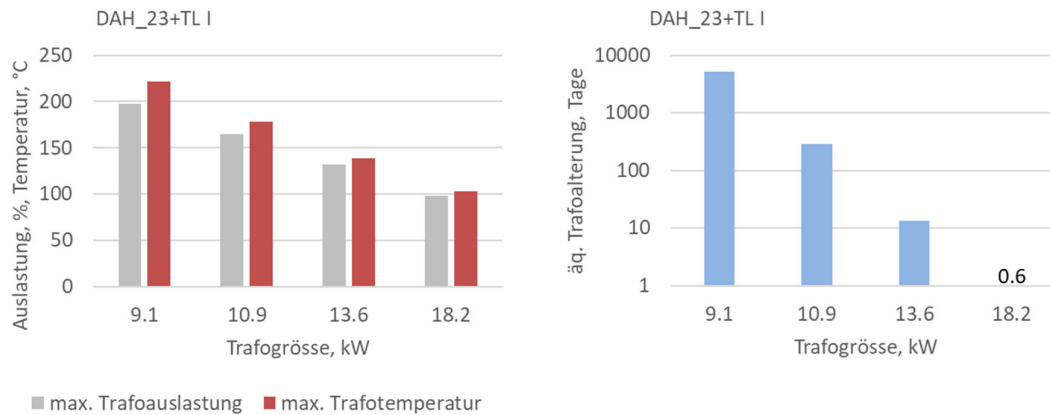
Abb. 23 Maximale Trafoauslastung und maximale Trafotemperatur (links) und äquivalenten Trafoalterung (rechts: Achtung logarithmische Skalierung) in Abhängigkeit von der Trafogröße für die Variante DAH_23+TL I.
