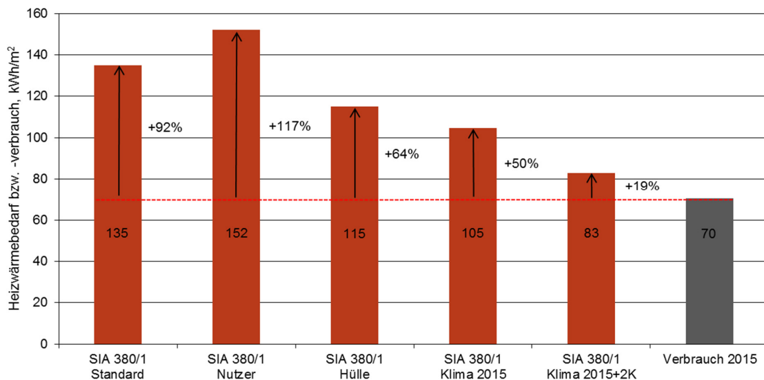
Bild 14 Bürogebäude: Vergleich Berechnung mit Standardeingabedaten ( HWB_{St} ) und mit messgestützten Eingabedaten ( HWB_{Kor} ) mit dem gemessenen HWV im Jahr 2015
