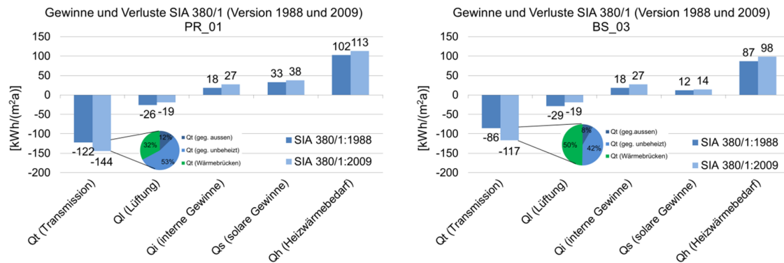
Bild 87 Berechnungsergebnisse Vergleich HWB St SIA 380/1 (Version 1988 und 2009) für die Gebäude PR_01 und BS_03
