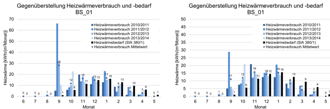
Bild 85 Links der mit ATD bereinigt HWV, rechts der mit HGT bereinigten HWV für das Gebäude BS_01.
