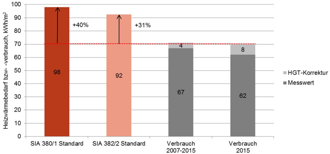
Bild 12 HWB St des Wohngebäudes berechnet mit Standardwerten und HWV gemessen mit Heizgradtag-Korrektur (HGT-Korrektur)
