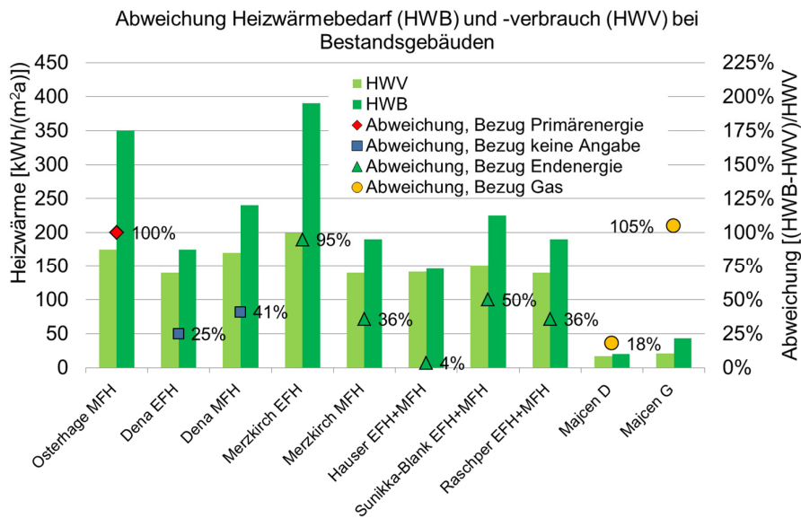
Bild 4 Unterschreitung des errechneten Heizenergiebedarfs durch den abgelesenen Verbrauch bei Bestandsgebäuden. Datenquelle: diverse Studien, der Name verweist immer auf den Erstautoren der Studie. Abkürzungen: EFH: Einfamilienhaus; MFH: Mehrfamilienhaus; D: Effizienzklasse D; G: Effizienzklasse G. Die Effizienzklassen gehen von A bis G, wobei A für sehr gut gedämmte Neubauten und G für sehr schlechte Bestandsgebäude steht. Ablesebeispiel: Abweichung + 25 %: Der Bedarf (B) liegt bei 175 kWh/m²a, der Verbrauch (V) liegt bei 140 kWh/m²a. (B - V)/V = 25\% Quellen: Osterhage [17]; Dena [21] der Dena Feldversuch wird in der genannten Quelle erwähnt, Merzkirch [19]; Hauser [26]; Sunikka-Blank [21], Raschper [22], Majcen [20], siehe hierzu auch den Kommentar bei Bild 5.
