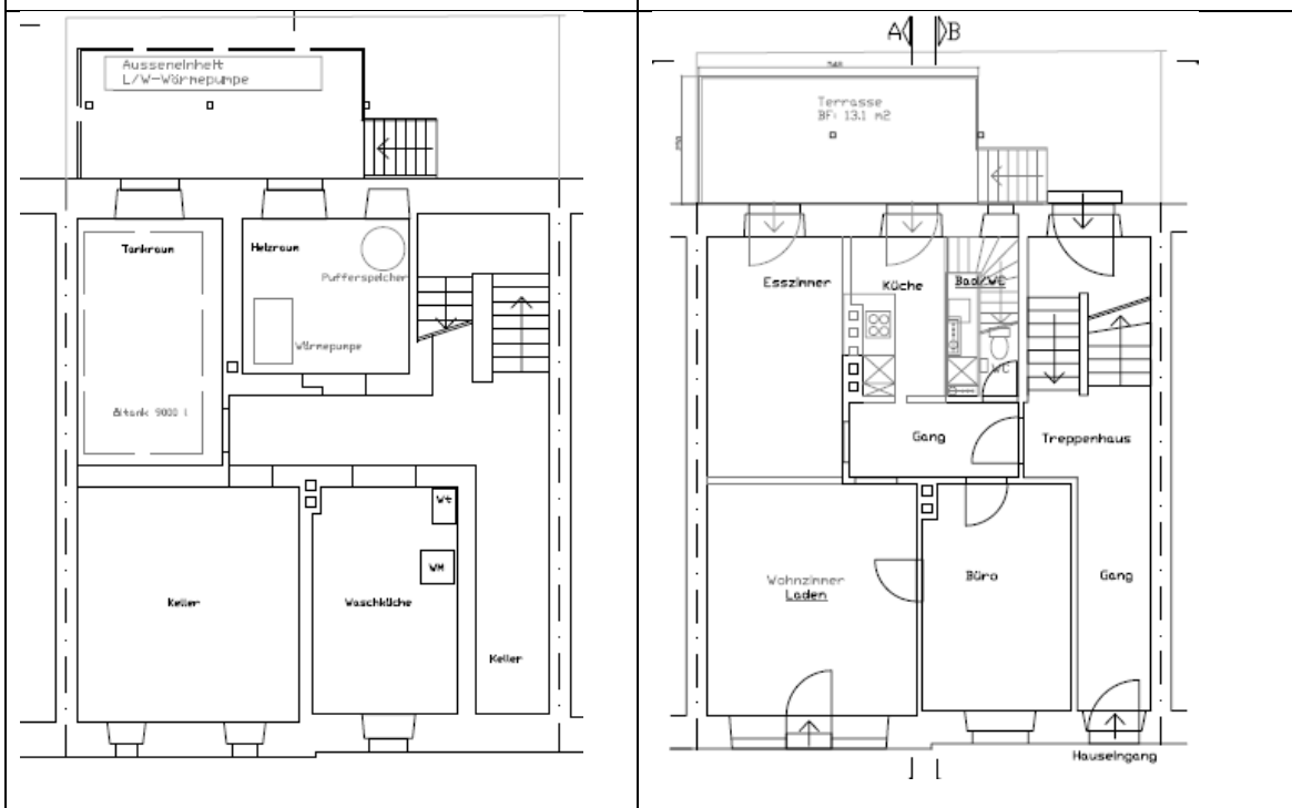
Bild 47 Grundriss UG
