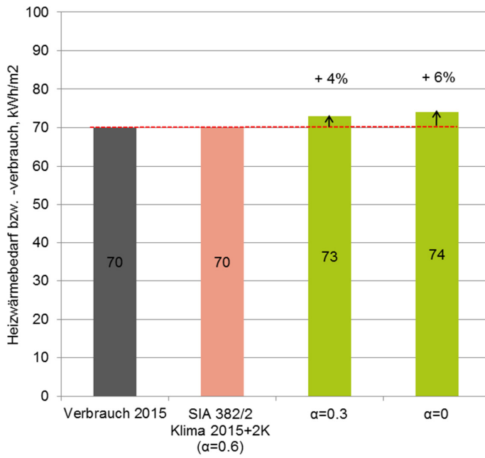
Bild 23 Einfluss Absorptionskoeffizient am Beispiel des Bürogebäudes. Vergleich HWV (grau) und HWB Kor (grün, rosa).
