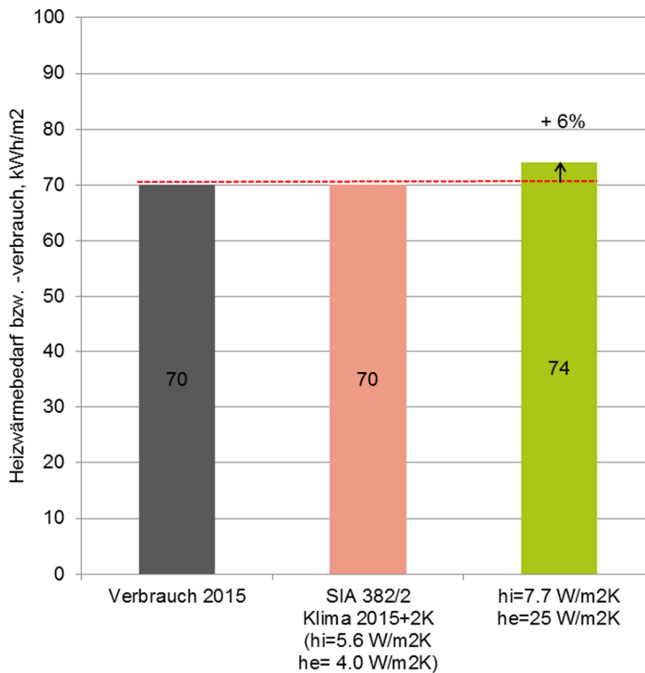
Bild 26 Einfluss Wärmeübergangskoeffizient am Beispiel des Bürogebäudes. Vergleich HWV (grau) und HWB Kor (grün, rosa).
