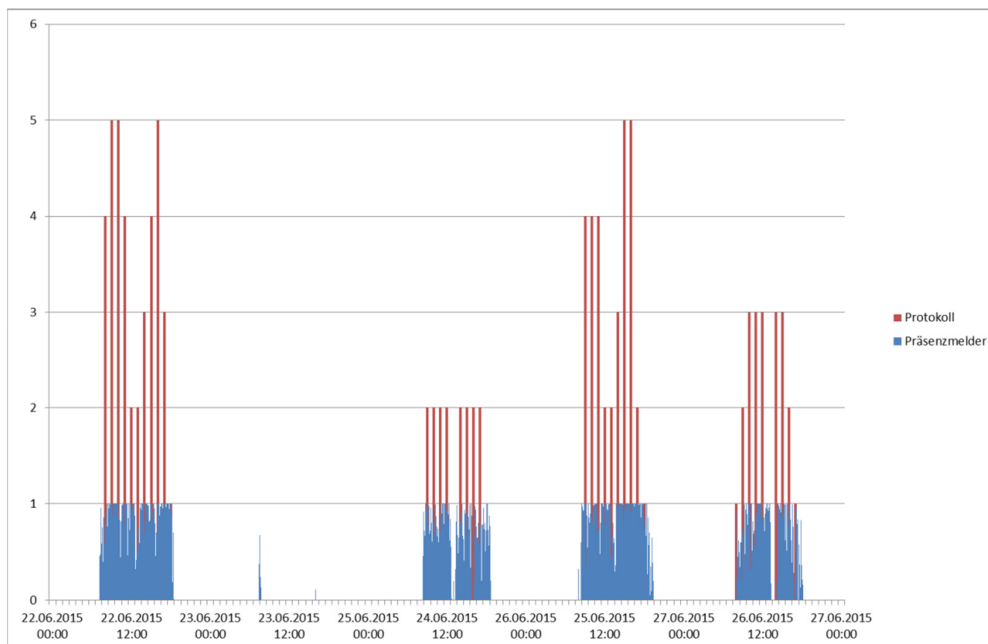
Bild 77 Personenpräsenz: Vergleich Bewegungsmelder und Anwesenheitsprotokoll
