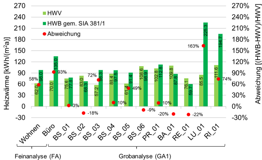
Bild 31 HWV und HWB_{St} (gem. SIA 380/1) für die beiden Gebäudegruppen FA und GA1. MFH: "Wohnen", BS_01, BS_02, BS_03, BS_04, BS_05, PR_01, BA_01 und RE_01. Das Gebäude BS_06 umfasst eine Mischnutzung mit Verkauf, Büro und Wohnen. EFH: LU_01 und RI_01 Flächenbezug: Energiebezugsfläche, A_E , gem. [32].
