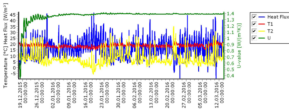
Bild 80 U-Wertmessung Westfassade Bürogebäude, 19.12.2015 – 12.03.2016
