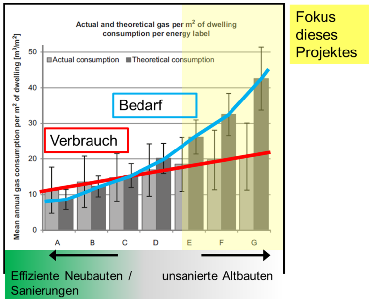
Bild 5 Verbrauch versus Bedarf bei Neubauten und Bestandsgebäuden. Grafik basiert auf: Gasbedarf versus Verbrauch von 200'000 EFH, MFH in den Niederlanden. Farbige Markierungen: die Verfasser. Anmerkung: Der jeweils verwendete Gaskesseltyp (konventioneller Kessel oder Brennwertkessel) werden in der niederländischen Berechnungssystematik sehr unterschiedlich bewertet, um so den Einsatz von Brennwertkesseln zu fördern [29]. In der Veröffentlichung wird nicht darauf eingegangen, wie diese Tatsache in der Untersuchung berücksichtigt wurde. Quelle: [20].
