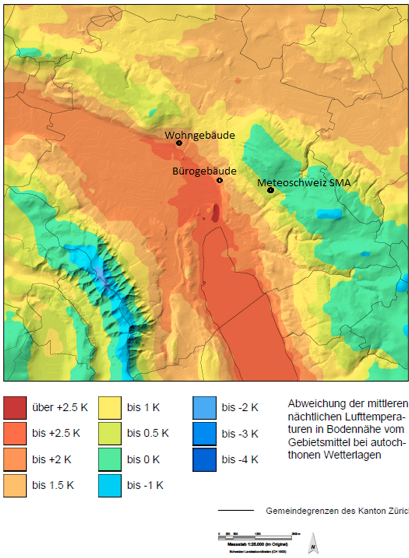
Bild 51 Nächtliche Wärmeinseln in Zürich. Quelle: [73]
