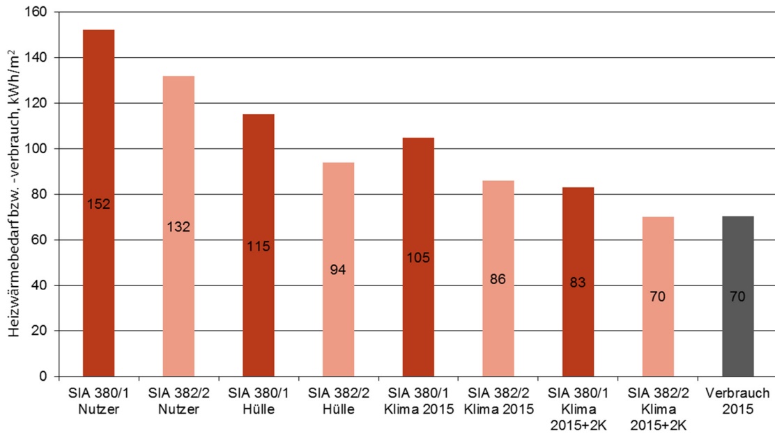
Bild 15 Bürogebäude: Vergleich der Ergebnisse HWB_{Kor} nach SIA 380/1:2009 (Monatsverfahren) und SIA 382/2:2011 (Stundenverfahren). Varianten von links nach rechts sind additiv (Änderungen jeweils zusätzlich).
