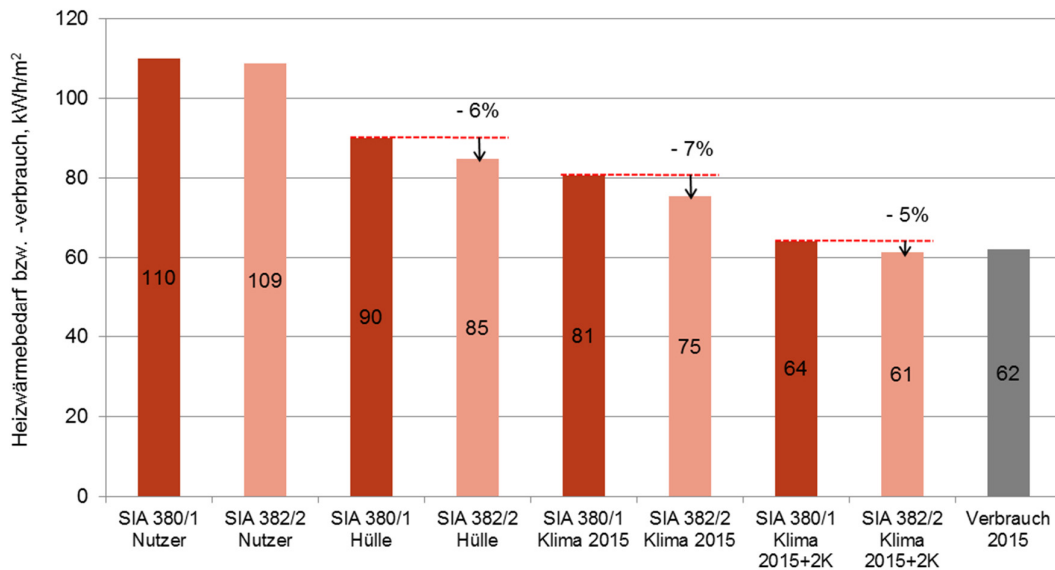
Bild 18 Vergleich der Ergebnisse HWB Kor nach SIA 380/1:2009 (Monatsverfahren) und SIA 382/2:2011 (Stundenverfahren)
