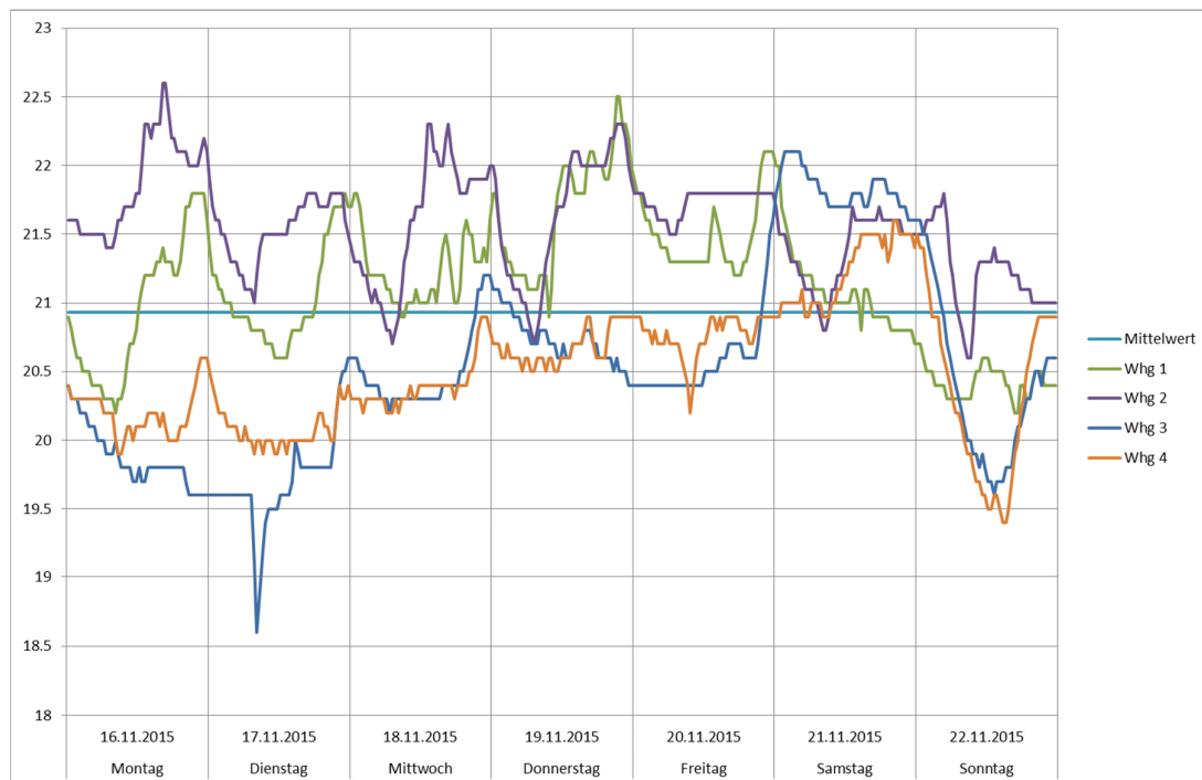
Bild 82 Raumlufttemperaturen MFH
