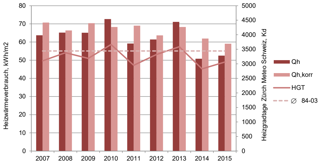
Bild 10 Heizwärmeverbrauch MFH Höggerstrasse; 2007 bis 2014: Abschätzung anhand Ölverbrauch 4 ; 2015: Messung Wärmehähler
