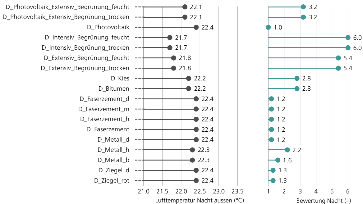
Abb. 18+19 Lufttemperatur (θ a ) Nacht aussen, 04:00 Uhr für die Dächer (links) und die Bewertung (rechts). Verwendete Abkürzungen: siehe Abkürzungsverzeichnis und Abb. 1 .
