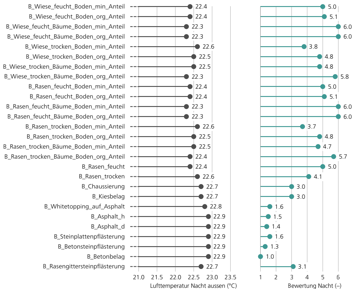
Abb. 16+17 Lufttemperatur (θ a ) Nacht aussen, 04:00 Uhr für die Böden (links) und die Bewertung (rechts). Verwendete Abkürzungen: siehe Abkürzungsverzeichnis und Abb. 1 .
