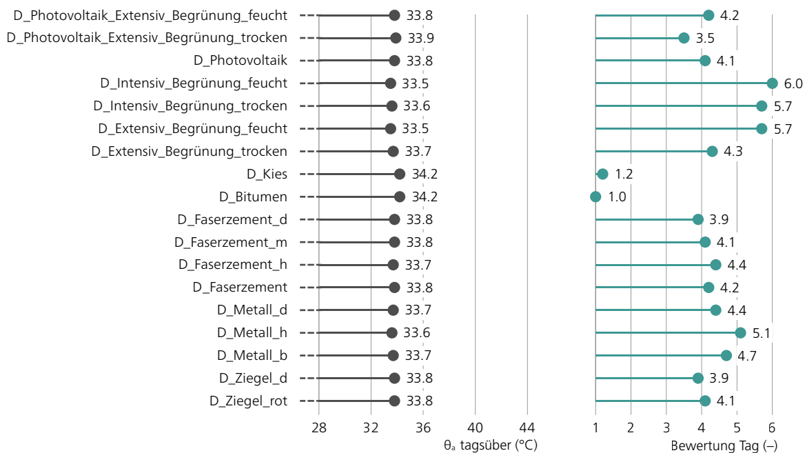
Abb. 12+13 Ergebnisse \theta_a tagsüber, 14:00 Uhr für die Dächer (links) und die Bewertung (rechts). Verwendete Abkürzungen: siehe Abkürzungsverzeichnis und Abb. 1.
