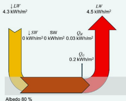
Abb. 66 Strahlungsbilanz «Albedo 80 %» von 21:00 bis 4:00 Uhr
