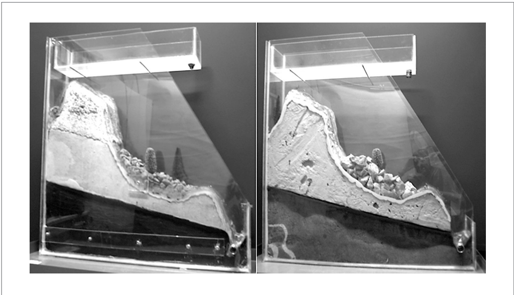
Abb. 2: Die beiden Quellenmodelle. Links: Porenquelle, rechts: Karstquelle.
