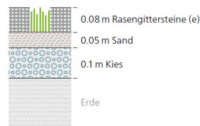
Aufbau
