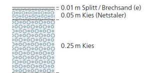
Aufbau
