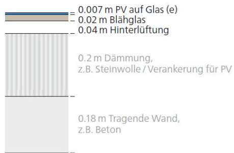
PV (hinterlüftet, Dämmung Steinwolle) → HF_Photovoltaik
