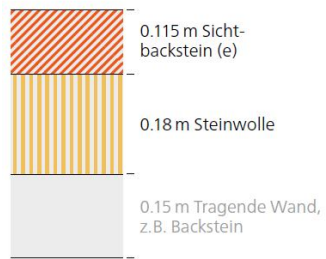
Zweischalenmauerwerk mit Kerndämmung, Sichtbackstein aussen → ZW_Zweischalenmauerwerk_Kerndämmung
