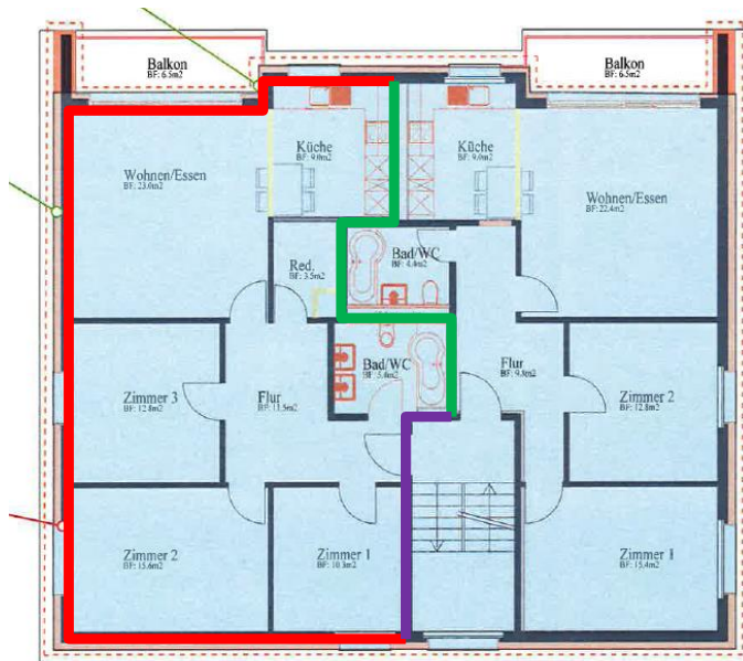
Figur 38 Randbedingungen für die Simulation rot = aussen, grün = adiat (Wand, Decke, Boden gegen Nachbarwohnung), lila = Treppenhaus, konstant 18°C
