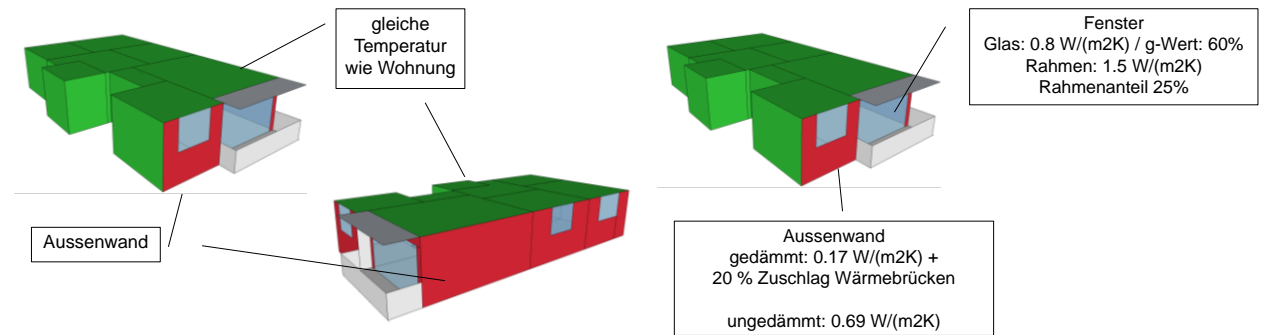
Figur 11: links: die thermischen Randbedingungen der Wohnung rechts: die U-Werte und g-Werte der Aussenbauteile
