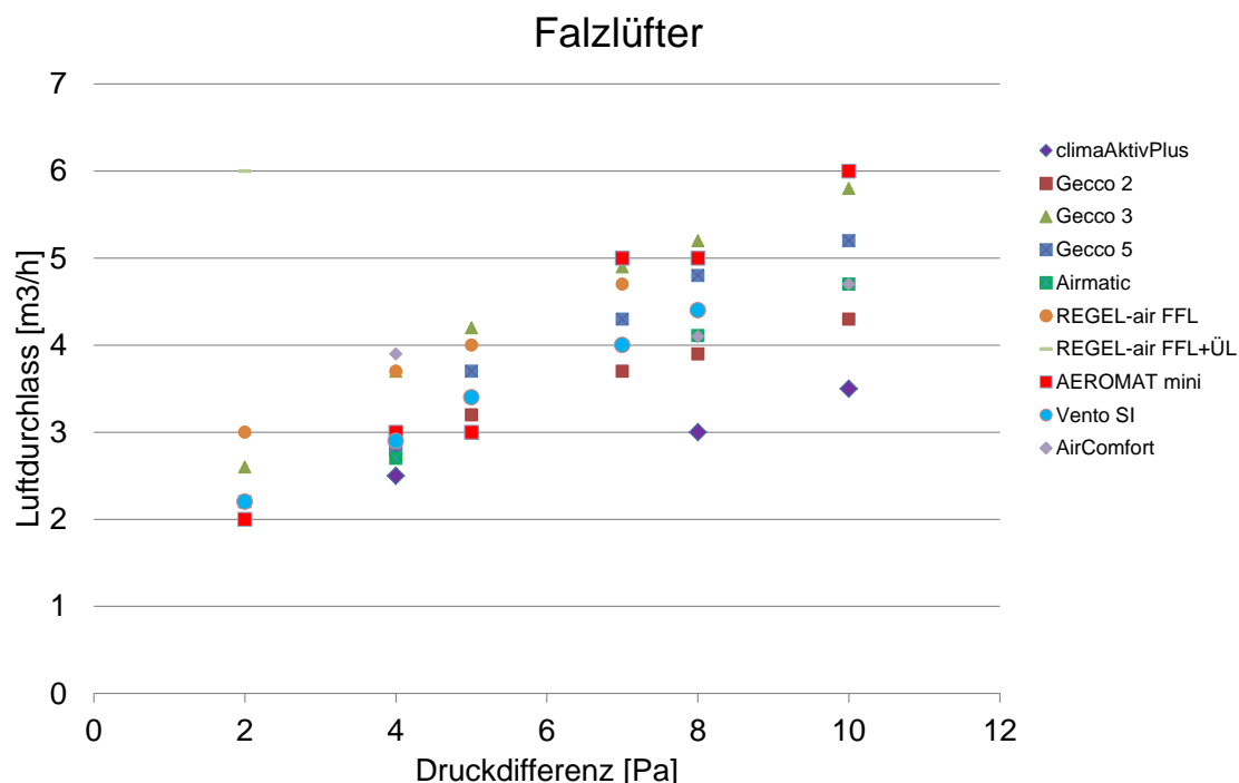
Figur 4: Leistungsdaten Falzlüfter
