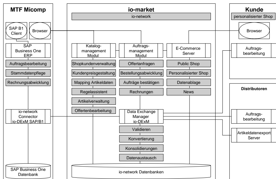
Abb. 5.4: Anwendungsübersicht MTF Micomp
