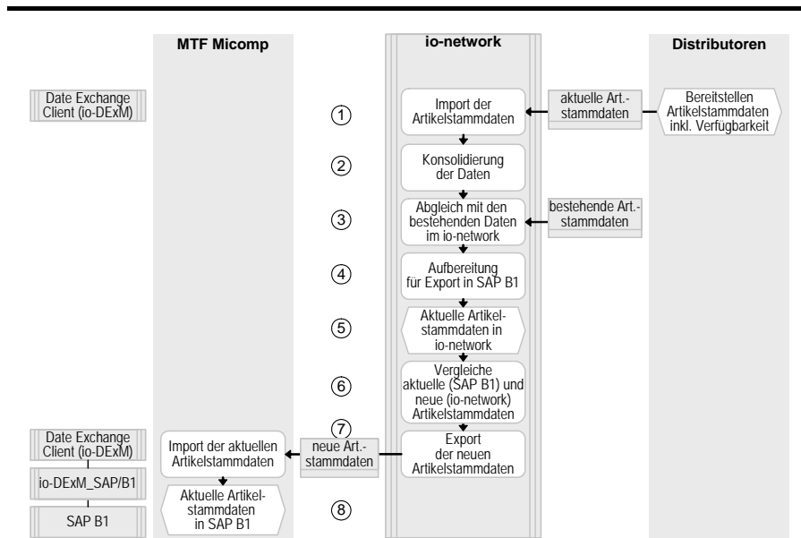
Abb. 5.2: Import der aktuellen Artikelstammdaten über das io-network
