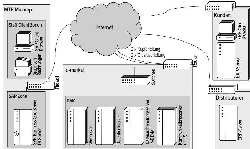
Abb. 5.5: Technische Sicht MTF Micomp
