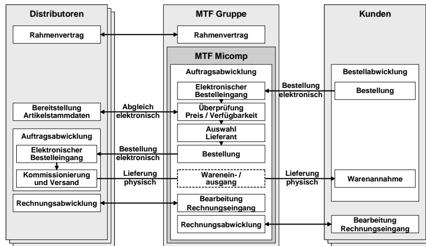
Abb. 5.1: Business Szenario: Auftragsabwicklung bei MTF Micomp
