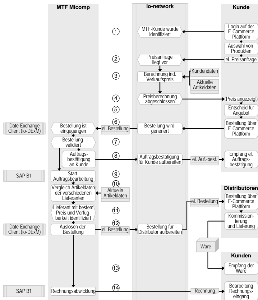
Abb. 5.3: Bestellprozess und Abläufe auf Seiten der MTF Micomp
